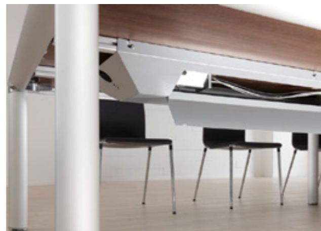
Vergaderruimtes met vast geïntegreerde technologie hebben bij P.A.L.M.A. een grote, eenvoudig toegankelijke kabelgoot. Hier zit alles op zijn plaats. De extra inzetbare Kabeltower ondersteunt daarbij de verticale kabelgeleiding op elegante wijze.
